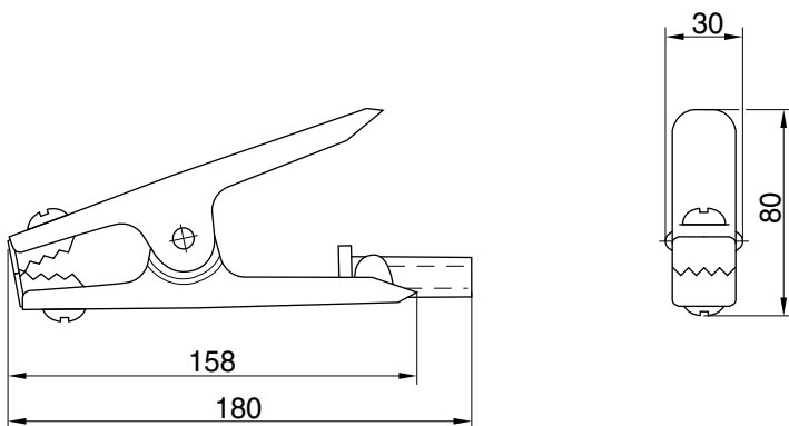
Abb. 19: Typ 70OK; maximale Zangen- öffnung 35 mm
