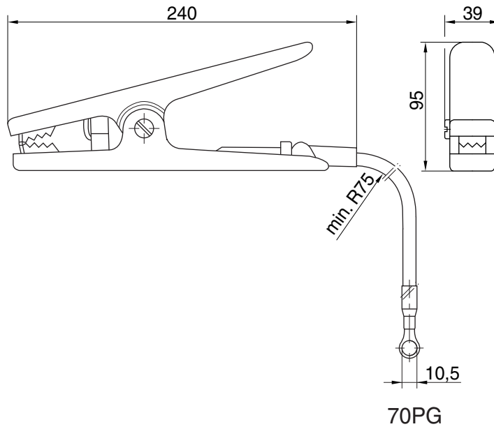
Abb. 16: Typ 70PG; maximale Zangen- öffnung 35 mm
